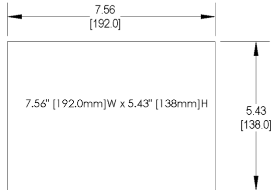
Cutout Dimensions
