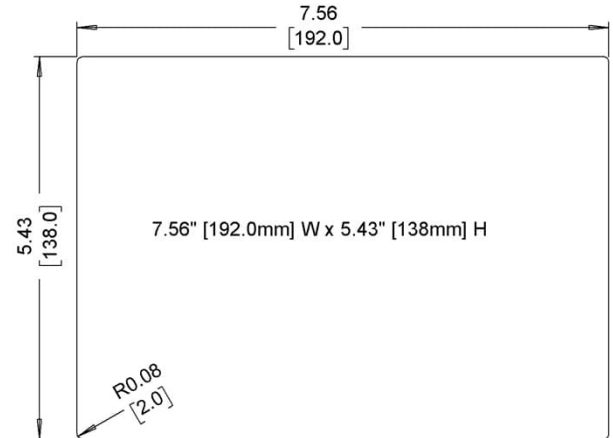
Cutout Dimensions
