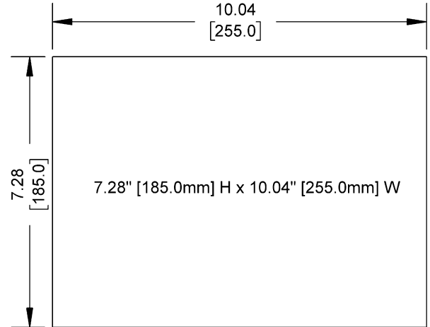
Cutout Dimensions
