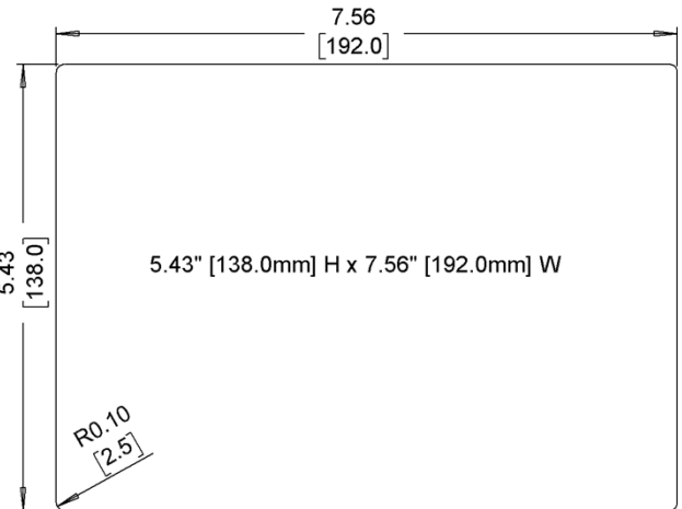
Cutout Dimensions
