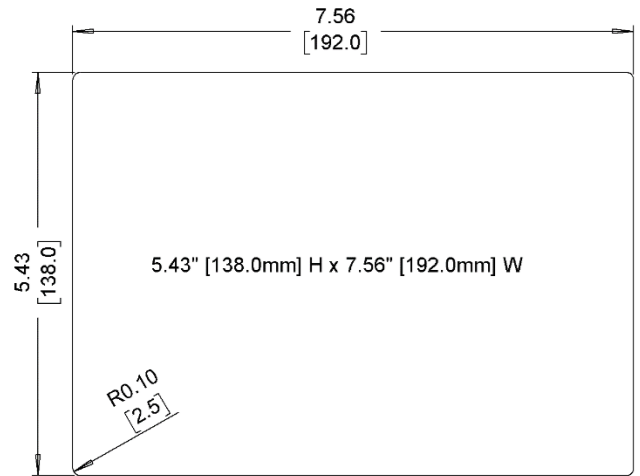
Cutout Dimensions
