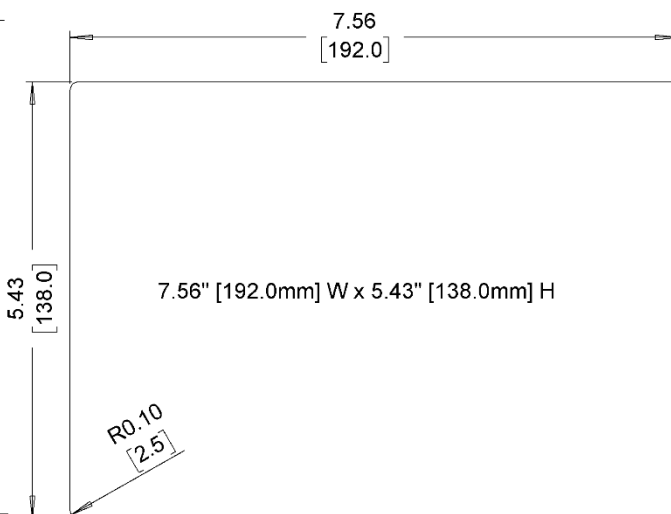
Cutout Dimensions
