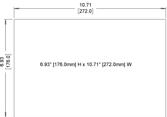
Cutout Dimensions
