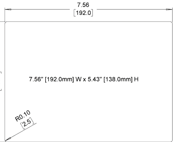
Cutout Dimensions
