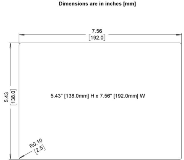
Cutout Dimensions
