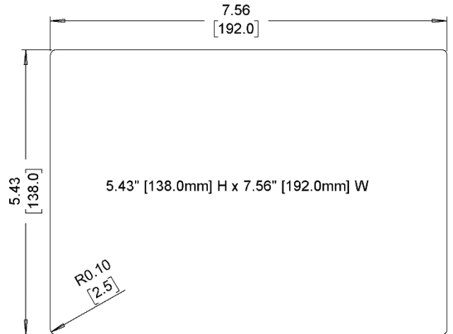
Cutout Dimensions
