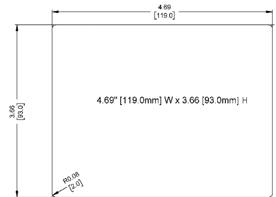
Cutout Dimensions
