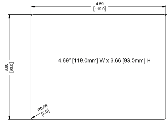
Cutout Dimensions
