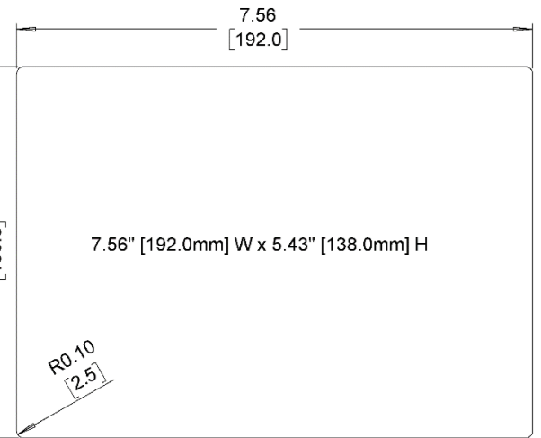
Cutout Dimensions
